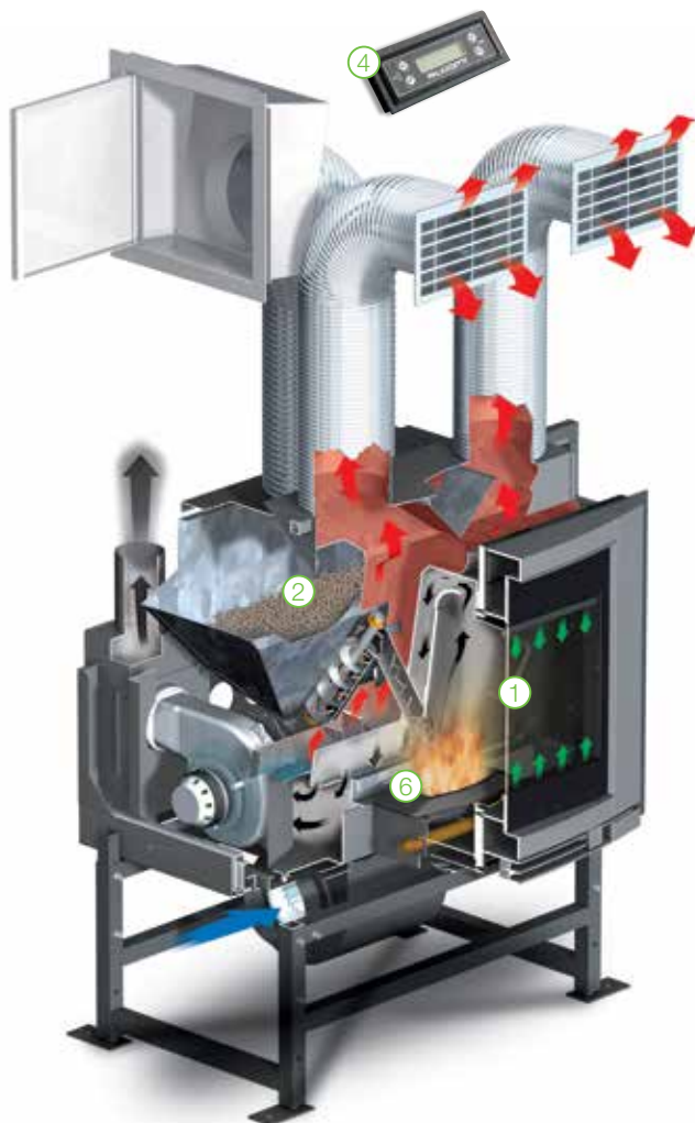
Ecofire da Inserimento canalizzabile.
